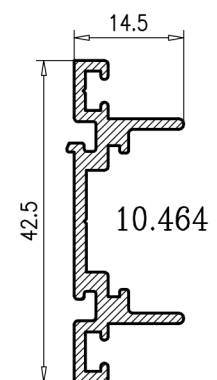
CIERRE MARCO
